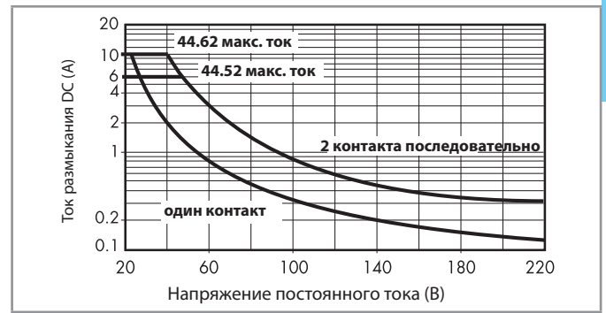
H 44 - Макс. отключающая способность DC1
