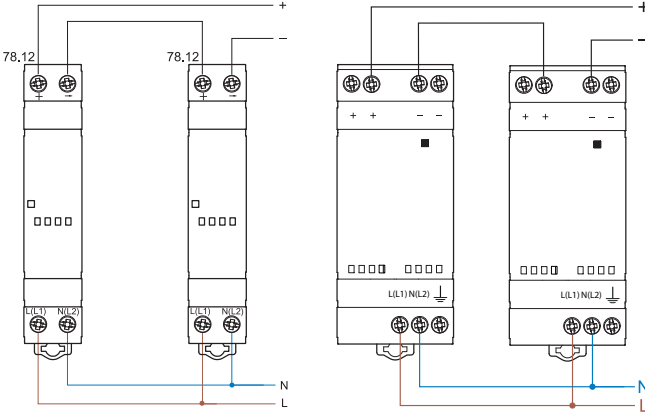
Последовательное соединение
