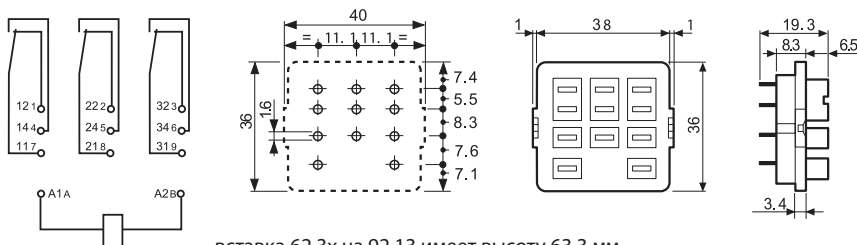
вставка 62.3х на 92.13 имеет высоту 63.3 мм
