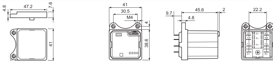
Адаптер крепления для типов 62.3x и 62.8x.xxxx.xxx9 (M4)
