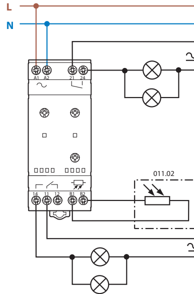
Тип 11.42
