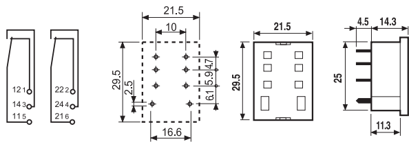
Вид со стороны выводов 96.12
