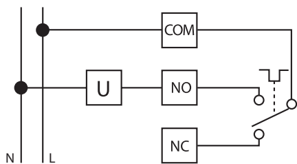
Схема подключения
