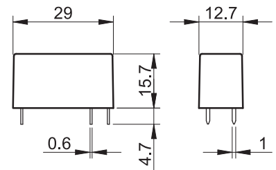
Тип 41.81-9024/41.81-8240
