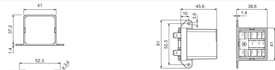
Фланцевый адаптер для типов 62.3x и 62.8x.xxxx.xxx9
