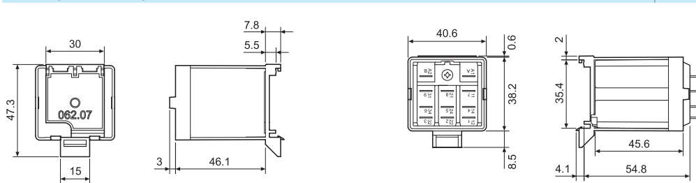
Адаптер для 35 мм рейки (EN 60715) для типов 62.3x и 62.8x.xxxx.xxx9
