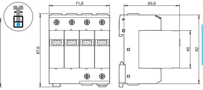
Тип 7P.26.9.420.1020
