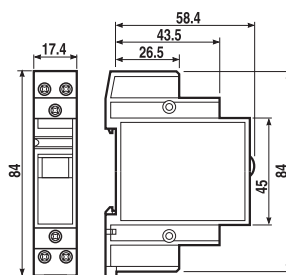
Тип 22.24
