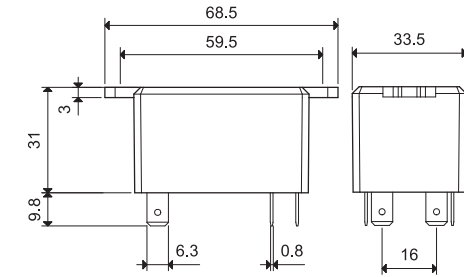
Тип 66.82-0300
