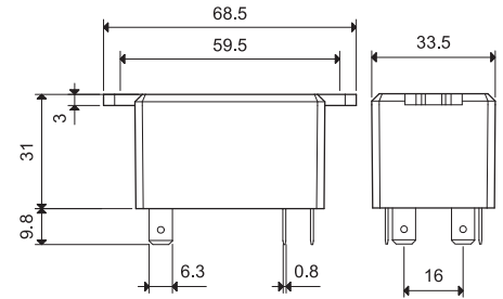
Тип 66.82-0600
