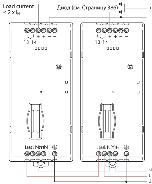
Параллельное подключение
