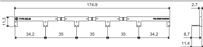
6-полюсная перемычка для Тип 22.34, ширина 35 мм 022.26 (синий)
