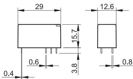
Тип 41.31/52/61
