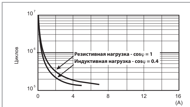
F 58 - Электрическая долговечность (AC) при ном. нагрузке Реле с 4 переключающими контактами
