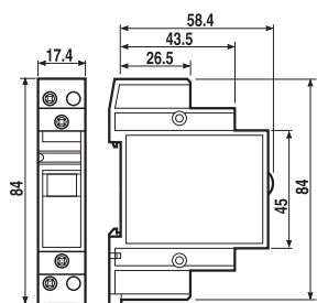
Тип 22.23
