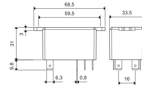
Тип 66.82
