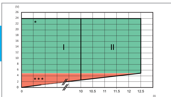
FB78-5 Зависимость выходного напряжение от выходного тока (78.2E)
